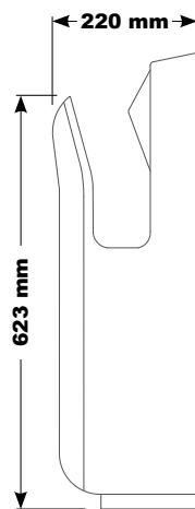
Vista lateral
