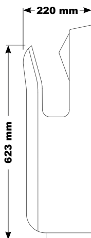
Seitenansicht
